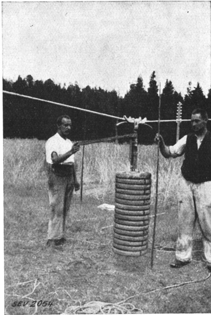
Fig. 4. Mitte der Spannweite S-T; das belastete Seil mit den Belastungsgewichten und der Auslösevorrichtung.
