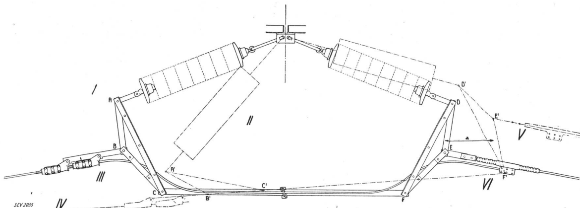
Fig. 5. 150-kV-Halbabspannung mit Trapez. Maßstab ca. 1:40. I Normalstellung. II Ausgelenkte Stellung. III Stromleiterseil durchgehend. IV Unbelastete Spannweite. V Belastete Spannweite. VI Variante mit Abspannmuffe, Stromleiterseil unterbrochen.
