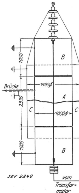
Fig. 3. Reuse zur Messung der Koronaverluste.
