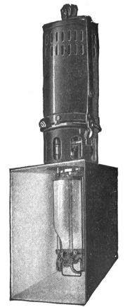
Fig. 4. Lichtpauz-Bogenlampe.
