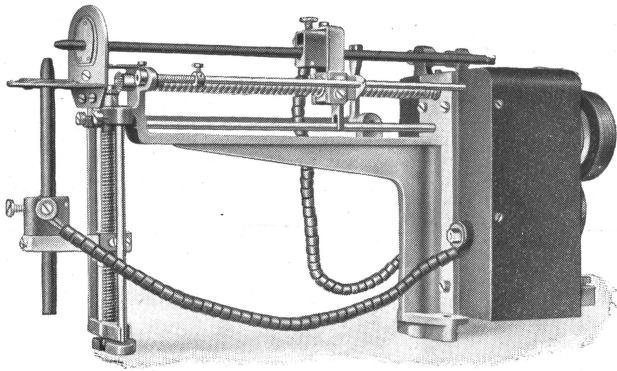
Fig. 6. Mikroprojektions-Bogenlampe.
