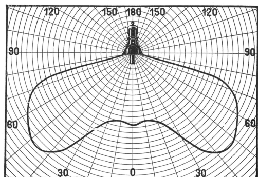
Fig. 1. Dia-Carbone-Bogenlampe mit tiefem Reflektor und Lichtausstrahlungskurve.
