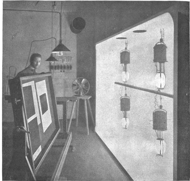
Fig. 7. Anwendung der Bogenlampe in der Reproduktionstechnik.
