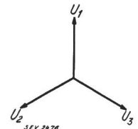
Fig. 17. Gegenläufiges Spannungssystem.
