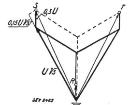
Fig. 6. Spannungserhöhung am Ende der Leitungsstrecke für einen Erdschluss am Anfang. Phase R hat Erdschluss.
