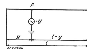
Fig. 5. Erdschluss in P . Unterteilung der Leitungsstrecke durch den Erdschluss.
