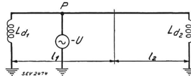
Fig. 15. Doppelseitig kompensierte Einfachleitung. Erdschluss in P.
