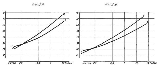
Fig. 7. Transformator A Transformator B Stationäre Wicklungs- und Oelübertemperaturen (°C) in Funktion der Belastung. 1 Oelerwärmung (obere Schicht). 2 Wicklungserwärmung (mittlere).
