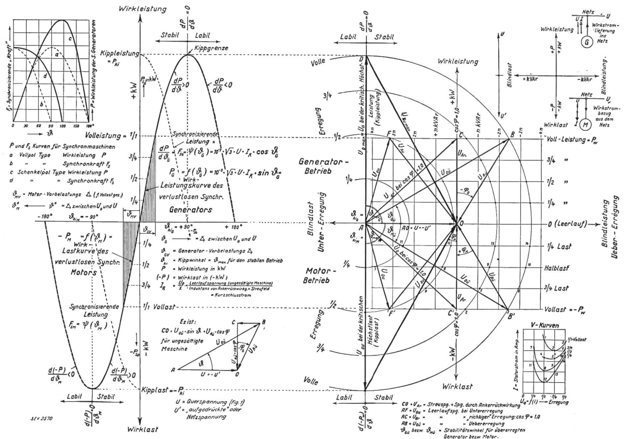
Fig. 3. Stabilitätsdiagramm und Leistungskurven einer verlustlosen und ungesättigten Vollpol-Synchronmaschine beim Motor- und Generatorbetrieb. (Anstatt F_{sg} und F_{sm} lies: P_{se} und P_{sm} ).
