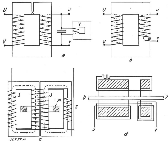
Fig. 27. Kunstschaltungen. a Nach Pfiffner. c Nach AEG. b Nach Wilson. d Nach Wellings und Mayo.
