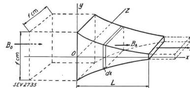
Fig. 28. Kernform zur Erzeugung der verlangten Kraftfluss-Magnetisierungskurve.
