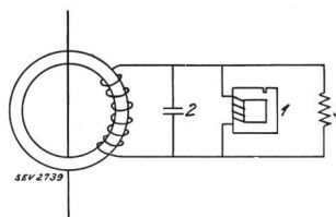
Fig. 34. Schaltungsschema des fehlerlosen Wandlers. 1 Drosselspule 2 Kapazität 3 Bürde
