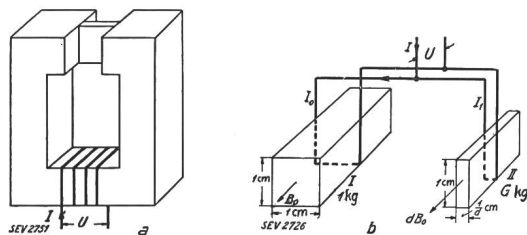
Fig. 20. b Ersatzschema des Kernes mit zwei Elementen. I Niedrige Liniendichte, Gewicht 1 kg. II Hohe Liniendichte, Gewicht G kg.
