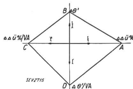
Fig. 9. Allgemeine Stromwandlercharakteristik.
