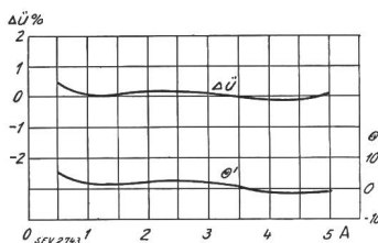
Fig. 38. Fehlerkurven ( \Delta \dot{u} \%_0 und \theta' ) des 200/5-A-Präzisionswandlers. D = 44 cm, H = 18 cm. Gewicht = 120 kg. Bürde = 0 bis 15 VA für \cos \varphi im Bereich von Fig. 39b
