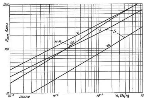
Fig. 3. Induktion ( B_{\max} ) in Funktion der Wirkleistung ( W ) und der Blindleistung ( VAr ) pro kg Silizium- resp. Nickel-Eisen ( Fe bzw. Ni-Fe ), bei 60 Per./s.
