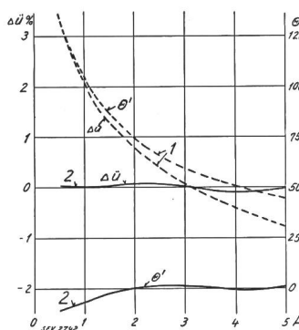
Fig. 37. Fehlerkurven ( \Delta \dot{u} \%_0 und \theta' ) des 400/5-A-Wandlers. D = 44 cm, H = 18 cm. Gewicht = 120 kg. Bürde = 0 bis 50 VA für \cos \varphi im Bereich von Fig. 39a. I Gewöhnlicher Wandler. II Präzisionswandler.
