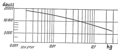
Fig. 25. Beziehung zwischen Liniendichte und Kerngewicht.
