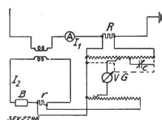
Fig. 42. Eichschaltung der Physikalisch-Technischen Reichsanstalt.
