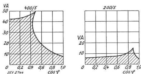
Fig. 39. 400/200/5-A-Wandler. Grenzen für Bürde und \cos \varphi .
