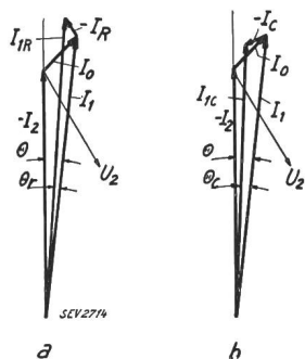
Fig. 8. a Fehlwinkelkorrektur mittels Widerstand. b Fehlwinkelkorrektur mittels Kapazität.
