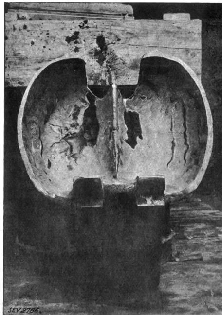
Fig. 2. Aube rechargée par le procédé Schoop, après trois semaines de service. Turbine Pelton: H = 260 \text{ m} ; P_e = 7360 \text{ kW} ; n = 300 \text{ t/m} .
