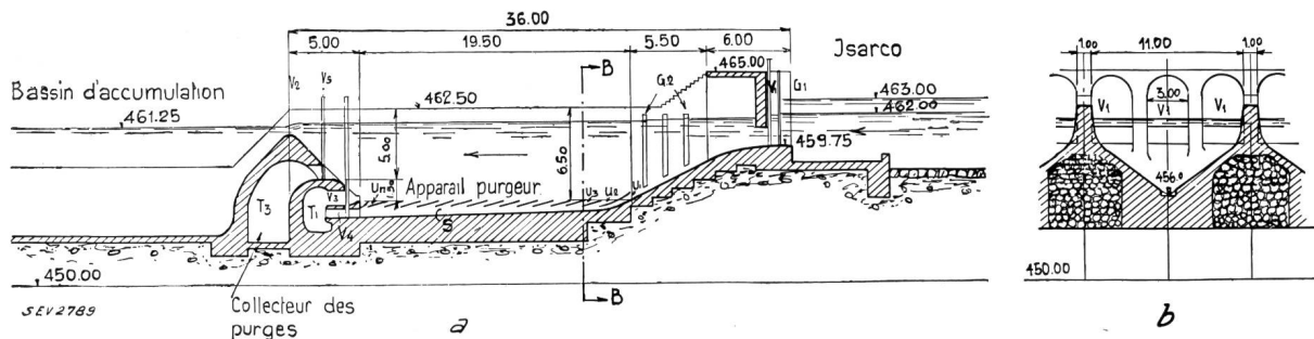
Fig. 5. Dessableur Dufour.
