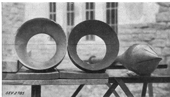
Fig. 1. Tuyères et pointeau usés par le sable. Turbine Pelton: H = 260 \text{ m} ; P_e = 7360 \text{ kW} ; n = 300 \text{ t/m} .
