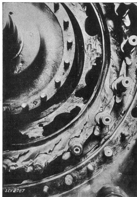
Fig. 3. Turbine Francis: H = 80 \text{ m} ; P_e = 2945 \text{ kW} ; n = 300 \text{ t/m} usée par le sable après trois ans de service; teneur moyenne de l'eau en alluvions 1,5 g/l.
