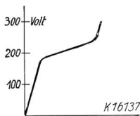
Fig. 4. Unterbrechungsvorgang. Zustand der Schaltstrecke während des Stromflusses.
