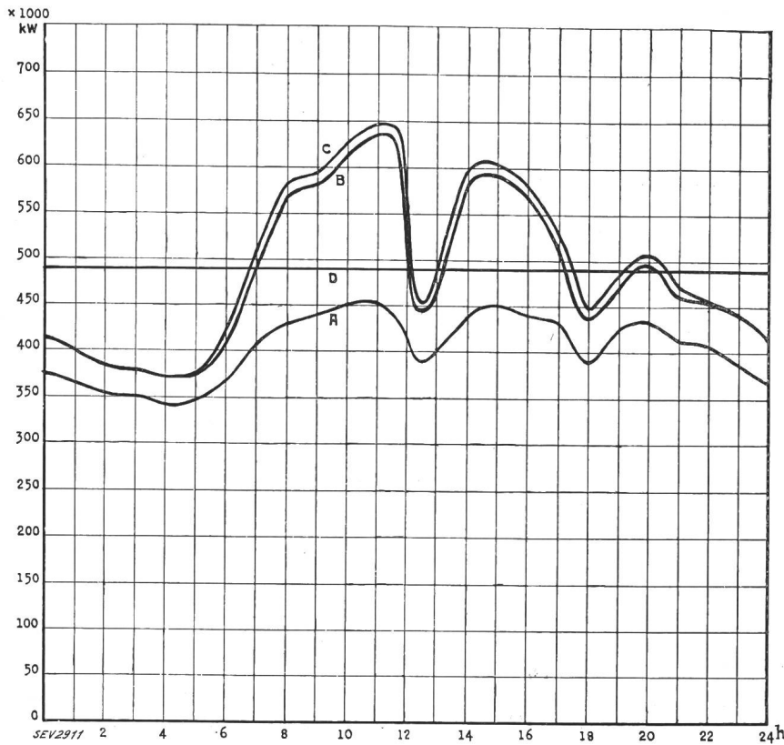
Diagramme journalier des puissances utilisées, mercredi le 17 septembre 1932.
