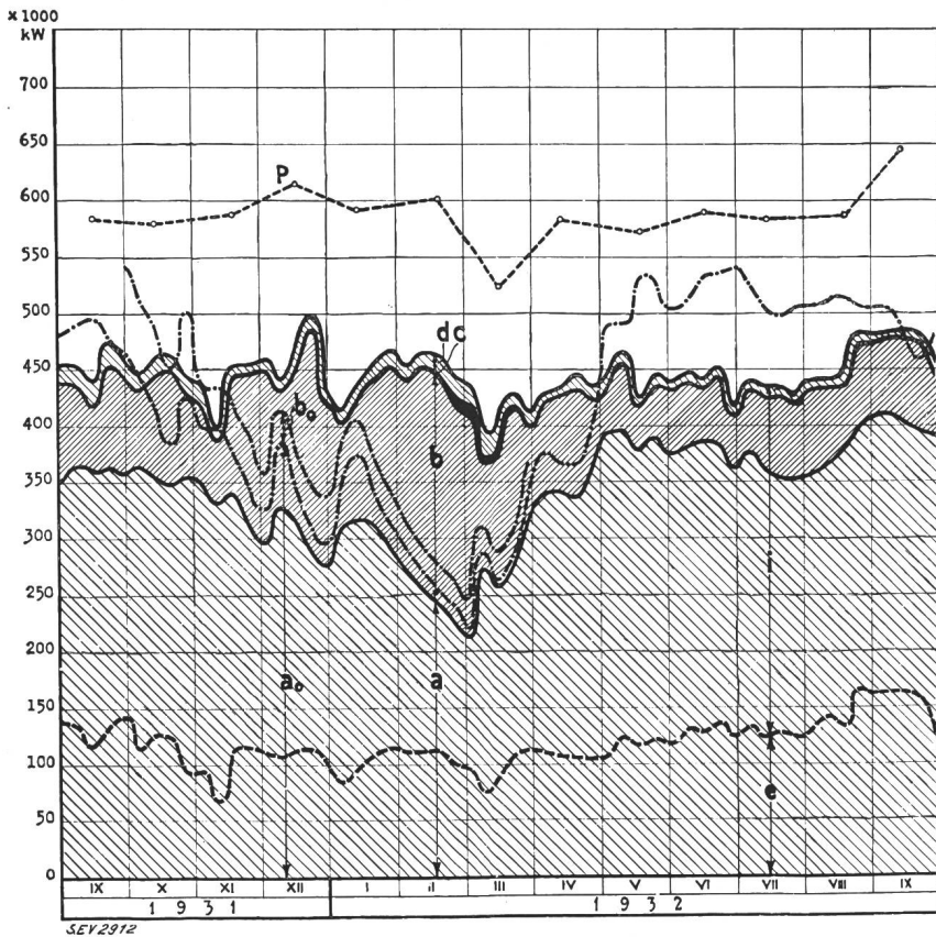
Diagramme annuel des puissances disponibles et utilisées, septembre 1931 à septembre 1932.
