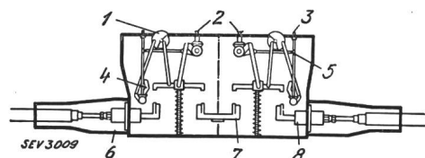
Fig. 3. Schema eines Kabelöltankens. 1 Anzeigevorrichtung. 2 Oelschalterbetätigungen. 3 Erdungsbetätigung. 4 Erdungsschalter. 5 Verriegelung. 6 Kabelendverschluss. 7 Sammelschiene. 8 Kabeldurchführung.
