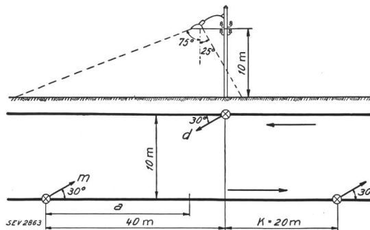
Fig. 16. Anordnung der Leuchten der Philora-Strassenbeleuchtung. m, d Projektionen der Reflektoraxen.
