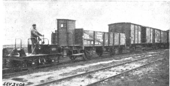
Fig. 6. Akkumulator-Schleppzug mit Batterie von 9 kWh.
