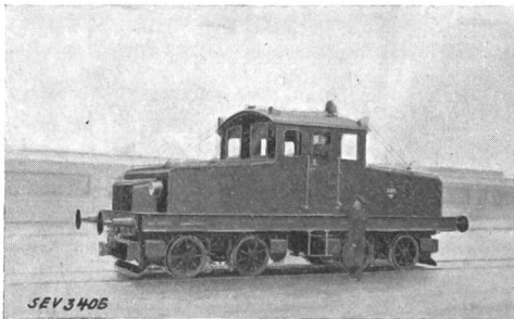
Fig. 4. Akkumulator-Verschiebe-Lokomotive mit Batterie von 110 kWh.
