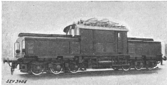
Fig. 3. Verschiebe-Lokomotive der Deutschen Reichsbahn für gemischten Akkumulator-Oberleitungsbetrieb (Gleichrichterumformung) mit Batterie von 357 kWh.
