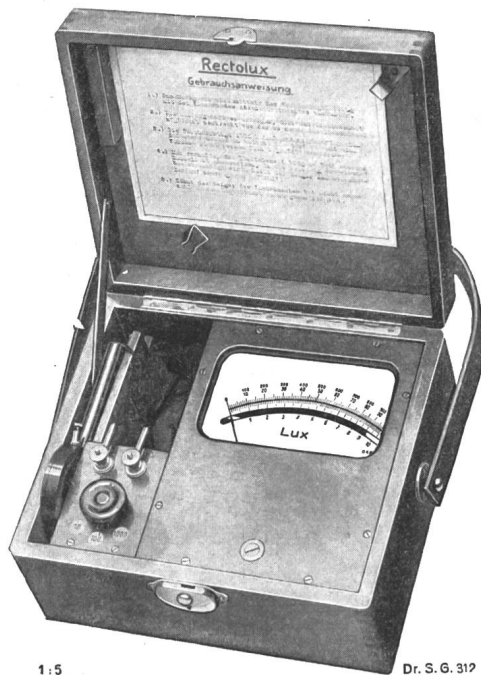
Fig. 9. Rektoluxmeter.
