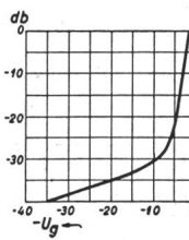
Fig. 4. Änderung des Verstärkungsgrades in Dezibel (db)
