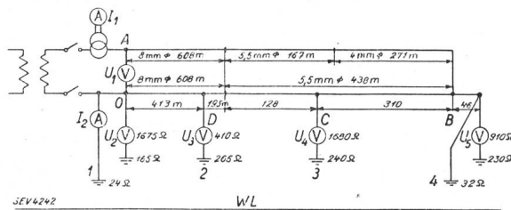
Fig. 56. 1 bis 4 Nummern der Erdungsstellen. WL Wasserleitung.
