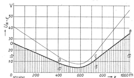
Fig. 57. Spannung ( U_{N-E} ) zwischen Nulleiter und Erde in Abhängigkeit der Entfernung ( x ) von der Transformatorstation. (Künstliche Erdungen am Anfang und Ende der Leitung. Fehlerstelle am Ende der Leitung.) Dickausgezogene Kurve: Phasenspannung = 137,5 V. Dünnausgezogene Kurve: Phasenspannung = 220 V. o Messpunkte.
