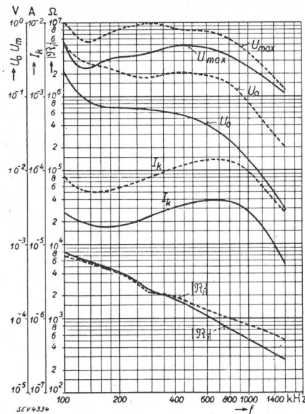
Fig. 5. Störungsdiagramm einer Heissluftdusche.
