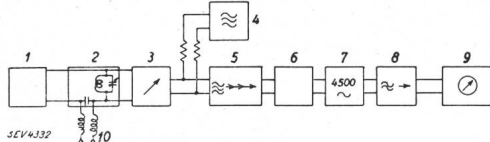
Fig. 3. Prinzip der Messapparatur.
