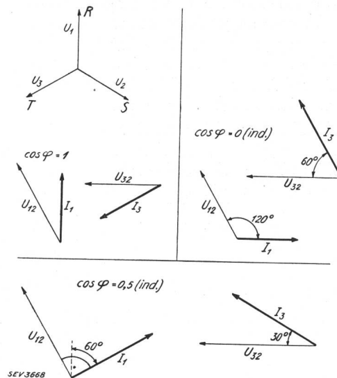
Fig. 8. Dreiphasenleistungsmessung nach der Zwei-Wattmeter-Methode.
