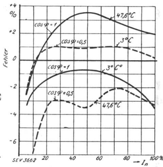
Fig. 2. Dreiphasenzähler Fabrikat B.
