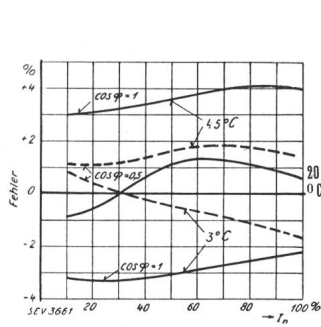
Fig. 1. Dreiphasenzähler Fabrikat A.
