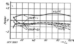
Fig. 5 (oben). Dreiphasenpräzisionszähler.
