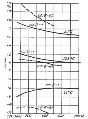
Fig. 6 (rechts). Registrierendes Wattmeter, Ferraris-Type.
