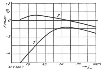
Fig. 7. Dreiphasenzähler, Einfluss der Reibung. 1 Fehlerkurve vor Revision, 2 Fehlerkurve nach Revision } \cos \varphi = 1
