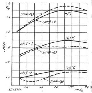
Fig. 4. Dreiphasenblindverbrauchzähler.
