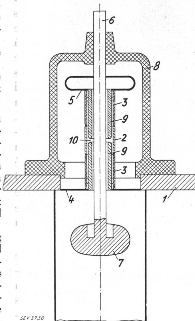
Fig. 1. Elektrodeneinführung.
