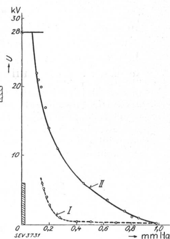
I Luft. II Quecksilberdampf.
