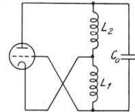
Fig. 6. Induktive Spannungsteilerschaltung.
