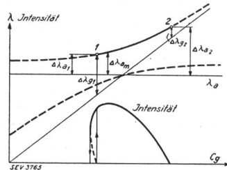
Fig. 7. Der Schwingbereich.
