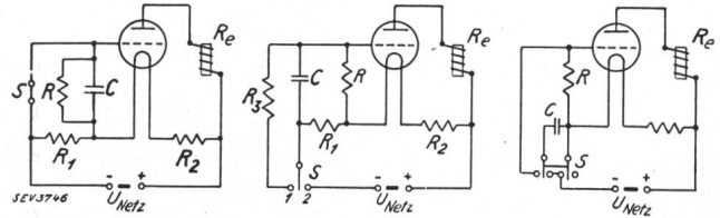
Fig. 1. Einfache Verzögerungsschaltung. Fig. 2. Schaltung mit nicht dauernd geheizter Röhre. Fig. 3. Schaltung für grosse Verzögerungen.
