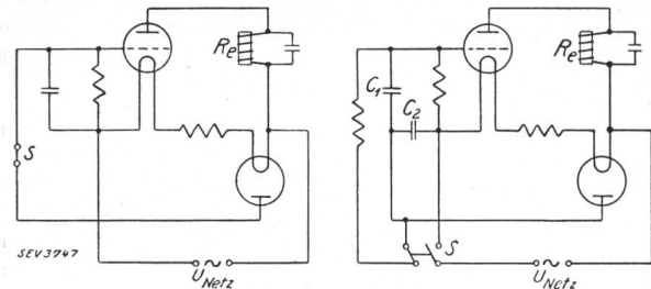
Fig. 4. Wechselstromschaltungen. Fig. 5.
