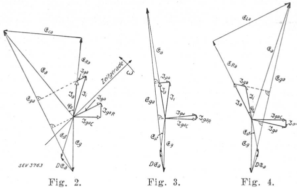
Fig. 2. Vektordiagramme.
