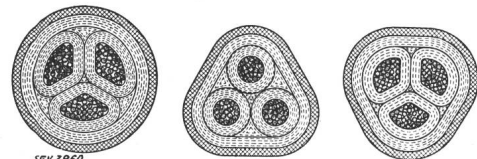
Fig. 1. Sektorkabel Fig. 2. SO-Kabel mit Gürtelisol. Fig. 3. T-SO-Kabel
