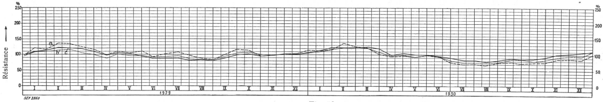
Fig. 5 b. Variation de la résistance à l'endroit de mesure N° 2, Affoltern a. A. Nature du terrain: Terre pierreuse (moraine de fond). Valeur moyenne de toutes les mesures 1929/30 = 100 %.
