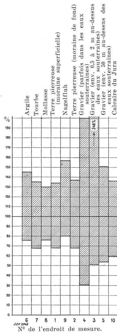
Fig. 4. Variations des résistances de terre de divers genres de terrains sous l'effet des conditions atmosphériques, déterminées à une profondeur de 0,5 à 0,7 m au-dessous du sol. Valeur moyenne tirée d'environ 50 mesures = 100 %.
