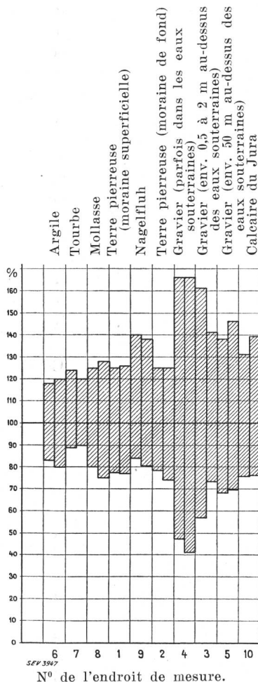
Fig. 3. Variations de la résistance spécifique de divers genres de terrains sous l'effet des conditions atmosphériques, déterminées à deux mises à la terre à une profondeur de 1 à 1,5 m au-dessous du sol. Valeur moyenne tirée d'environ 50 mesures = 100 %.
