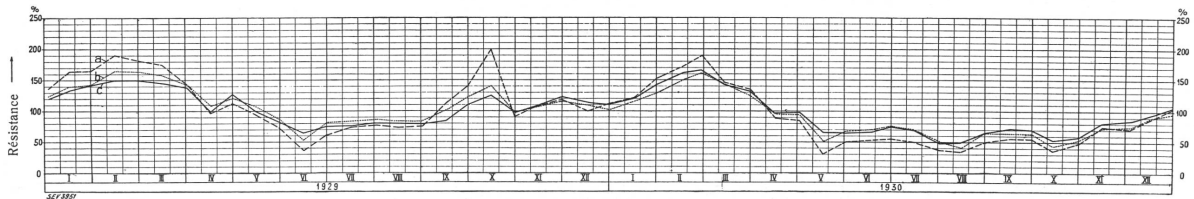
Fig. 5 c. Variation de la résistance à l'endroit de mesure N° 4, Dietikon. Nature du terrain: Gravier noyé parfois dans les eaux souterraines. Valeur moyenne de toutes les mesures 1929/30 = 100 %.
