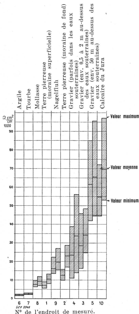
Fig. 2. Résistances spécifiques de divers genres de terrains, déterminées au cours de deux années à deux mises à la terre à une profondeur de 1 à 1,5 m au-dessous du sol.
