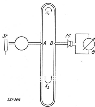
Fig. 2. Apparat von Quincke.
