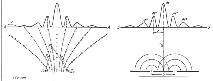
Fig. 5. Interferenzfeld zweier Kreiswellen.
