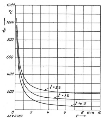
Fig. 3. Stationäre Temperaturverteilung nach Gl. (22) für verschiedene Zeiten.
