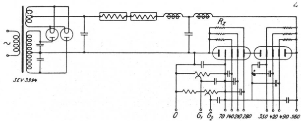
Fig. 4. Stabilisiertes Netzanschlussgerät.
