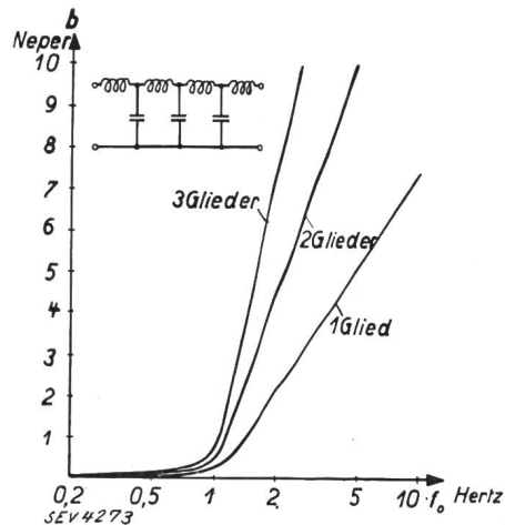
Fig. 9. Spulenkette und ihre Dämpfungseigenschaft.
