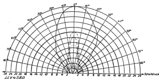
Fig. 16. Polardiagramm eines Trichterlautsprechers mit geradem Trichter.
