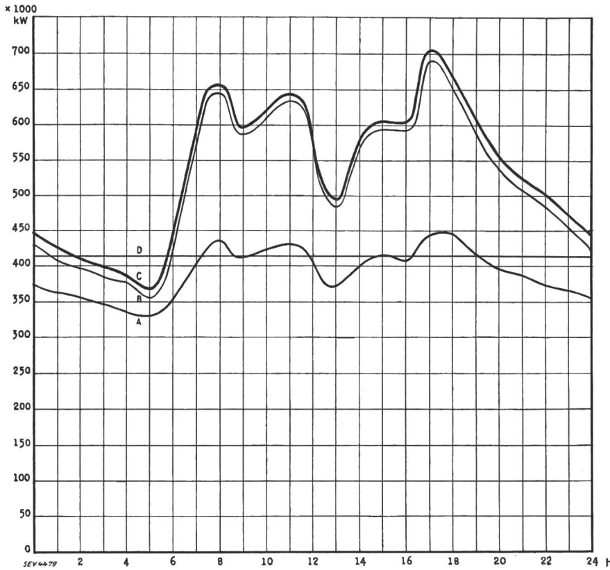
Diagramme de charge journalier du mercredi 12 décembre 1934.
