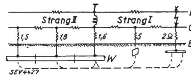
Fig. 11. Normalspannungsnetz mit gemischter Erdung. x Fehlerstelle; T Transformator.
