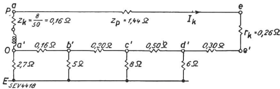
Fig. 2. Schematischer Netzplan.
