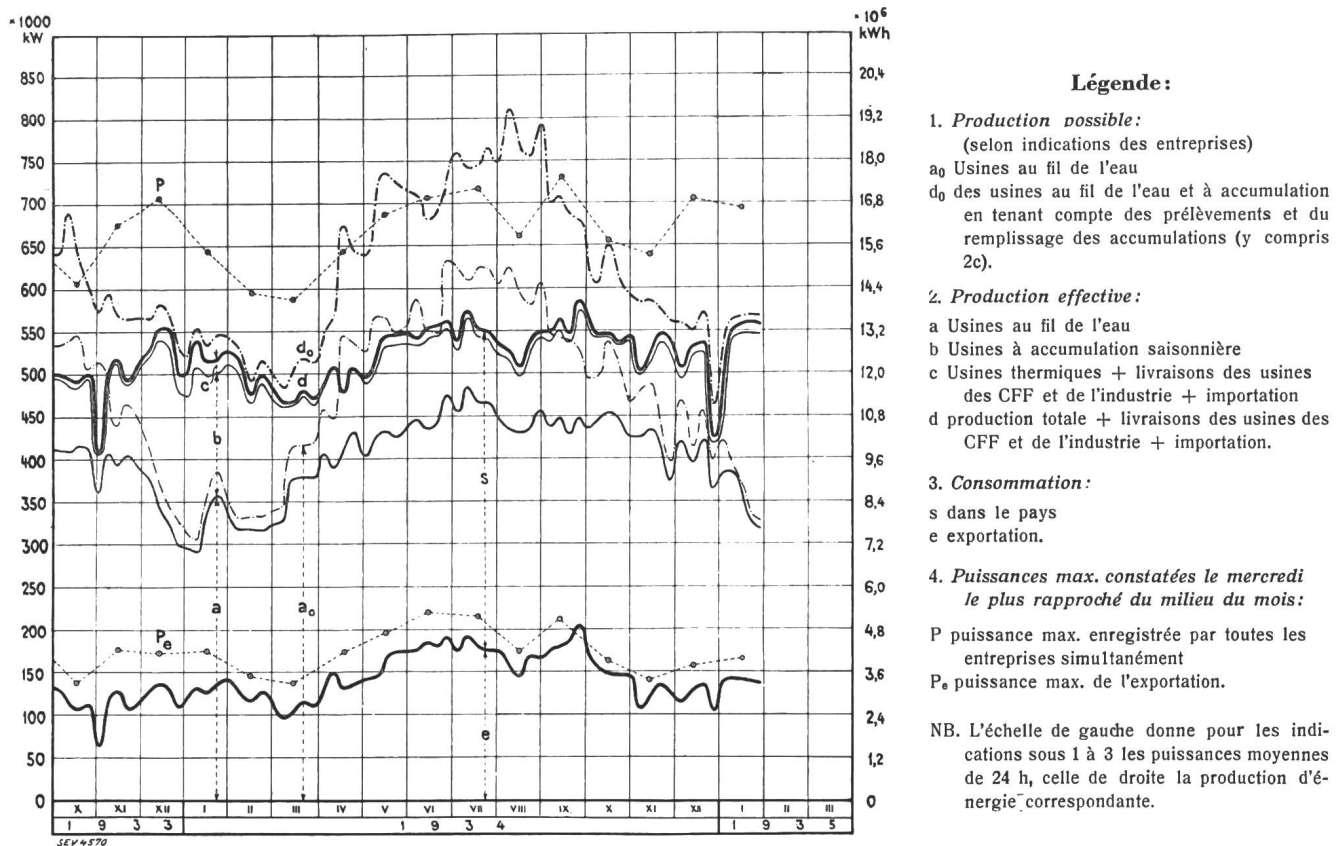
Diagramme annuel des puissances disponibles et utilisées, octobre 1933 à janvier 1935.
