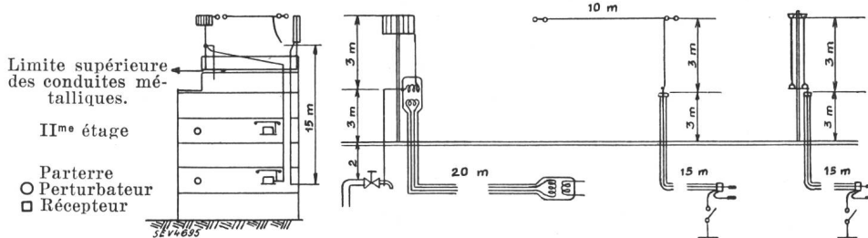
Fig. 3b. Bâtiment où les mesures B ont été effectuées. S Câble à écran (Silberantenne).
