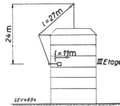
Fig. 3. Disposition des antennes A.
