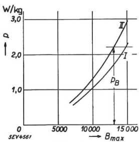
Fig. 1. Verlustkurven. I 1,05-Watt-Blech. II 1,3-Watt-Blech.
