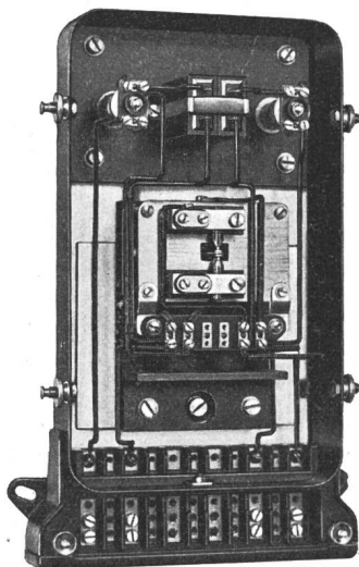
Fig. 7. Relais émetteur (L & G).
