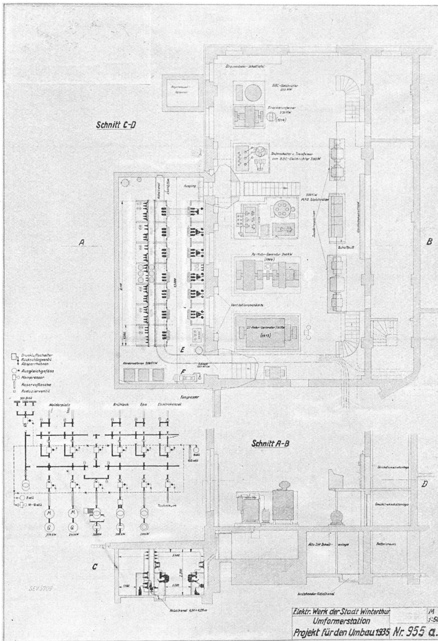
Fig. 8. Umformerstation, Umbauprojekt.
