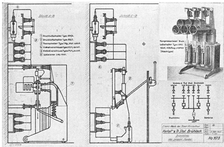
Fig. 1. Projekt für den Umbau der Schaltstation Brühleck.
