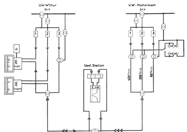
Fig. 13. Prinzipschema der Fernmessanlage.
