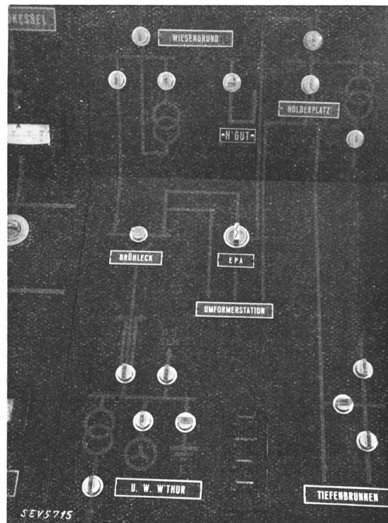
Fig. 16. Fernmeldeanlage: Rückmeldeschema auf dem Schaltpult.
