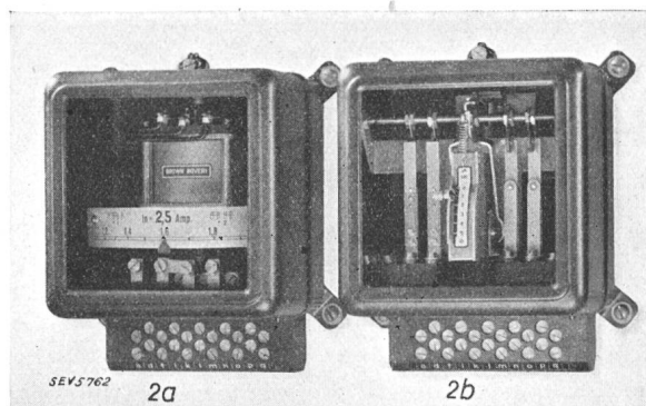
Fig. 2. Separates Strom- und Zeitrelais. 2a Momentan wirkendes Ueberstromrelais mit 3/10 VA Eigenverbrauch. 2b Zeitrelais.
