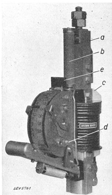
Fig. 1. Hochstromsicheres Primärrelais. a Isolation des oberen Anschlusses. b Ueberbrückungswiderstand gegen Sprungwellen. c Spulenabstützungen. d Einstellbare Grenzstromauslösung.
