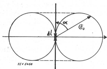
Fig. 1. Strahlungscharakteristik eines geraden Stromelementes.
