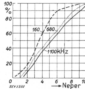
Fig. 5. Zusammenstellung aller Messungen der unsymmetrischen Komponente.
