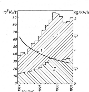
Fig. 1. Thermische (I) und hydraulische (II) Energieerzeugung. Kurve I: Spezifischer Verbrauch der thermischen Werke an Kohle (7200 kcal/kg) in kg/kWh.
