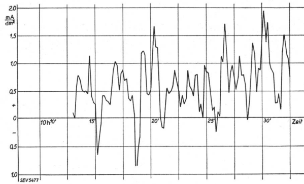
Fig. 4. Sondennmessungen am Rohr von 25 mm \varnothing .
