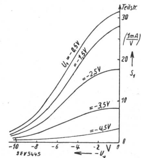
Fig. 5. Steilheit S_1 der Anodenstromkennlinien I_a = f(U_1) der 'Misch-Hexode' Valvo X 4122 in Abhängigkeit der Gittervorspannung U_4 .
