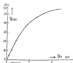
Fig. 9. Amplitude der Zwischenfrequenz u_{az} in Abhängigkeit der Wechselspannung u_1 . U_1 = -1,5 V; U_4 = -4 V; u_4 = 2 V.
