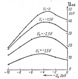
Fig. 8b. Amplitude der Zwischenfrequenz u_{az} in Abhängigkeit der Gittervorspannung U_4 und U_1 ; u_1 = 0,9 V; u_4 = 2 V.
