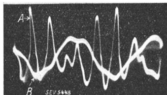
Fig. 7d. Resultierende Anodenwechselspannung u . Kurve B Zwischenfrequenz U_1 = -1,5 V; U_4 = -4 V; u_1 = 0,8 V; u_4 = 4 V.
