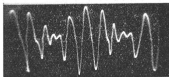
Fig. 7c. Schwungskomponente der Anodenwechselspannung. S_1 \cdot R_{a1} \cdot u_1 \sin \omega_1 \cdot t + S_4 \cdot R_{a4} \cdot u_4 \sin \omega_2 \cdot t ; U_1 = -1,5 V; U_4 = -4 V; u_1 = 0,8 V; u_4 = 4 V.
