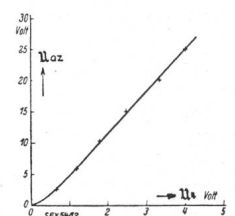
Fig. 10. Amplitude der Zwischenfrequenz u_{az} in Abhängigkeit der Wechselspannung u_4 . U_1 = -1,5 V; U_4 = -4 V; u_1 = 0,2 V.
