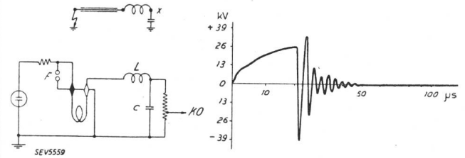
Fig. 6. Oscillation aux bornes d'une petite capacité C \approx 5 \cdot 10^{-10} \text{ F} (représentant un petit poste de transformateurs) en série avec une self, L = 0,6 \text{ m H} , branchée à l'extrémité de 100 m de câble.
