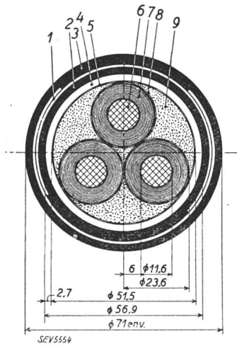
Fig. 1. Section droite d'un câble 3 \times 80 \text{ mm}^2 \text{ H. } 20 \text{ kV. Type C1. 1 Armure; 2 Feuille d'as 1 mm. 2,3 Jute asphalté. 4 Plomb. 5 Toile métallisée. 6 Conducteur en cuivre. 7 Isolation en papier imprégné. 8 Papier métallisé. 9 Bourrage.
