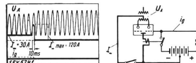
Fig. 3. Gesteuerter Hochspannungs-Gross-Mutator 13 kV, 30 A. Abschalten von Kurzschlüssen. (Abschalten durch Gitter ohne Drosselspule.)
