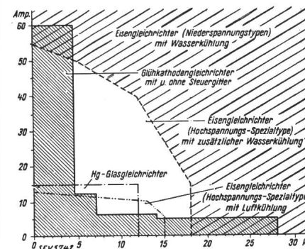
Fig. 4. Grenzleistungen der verschiedenen Mutatorarten. (Für Sechschphasenschaltung, bzw. Dreiphasen-Graetzschaltung der Mutatoren.)
