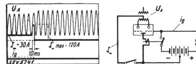
Fig. 3. Gesteuerter Hochspannungs-Grossmutator 13 kV, 30 A. Abschalten von Kurzschlüssen. (Abschalten durch Gitter ohne Drosselspule.)
