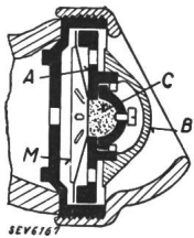
Fig. 3. USA-Mikrophon.
