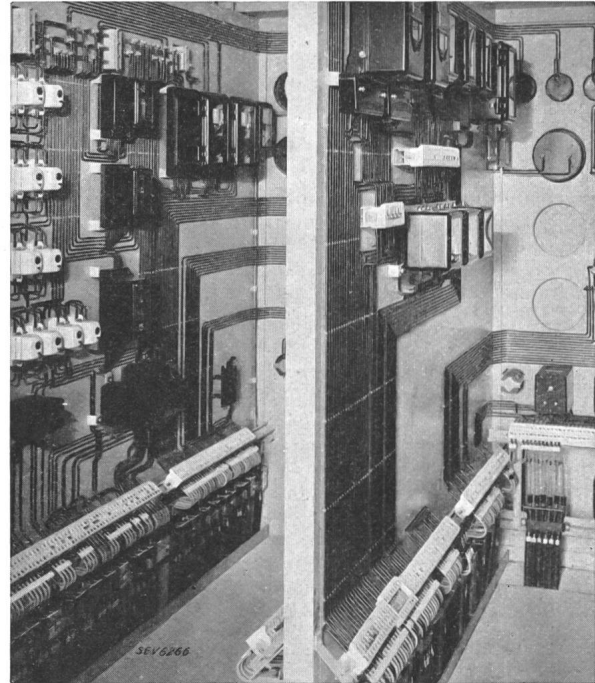
Fig. 1. Exemple de câblage d'une installation.
