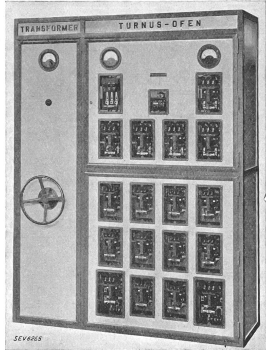
Fig. 4. Hauptverteilt-Tableau mit Schützensteuerung (Frontdeckel der Apparate entfernt).
