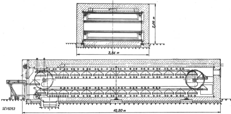
Fig. 3. Längs- und Querschnitt des Turnusofens «Tu. 3,8C».
