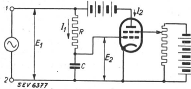
Fig. 2. Grundsätzliches Schema einer Röhrenschialtung, die als scheinbare Selbstinduktion wirkt.
