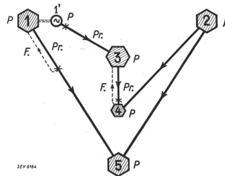
Fig. 21. Einfache Kupplung mehrerer Netze. P Leistungsregulierung. Pr Lieferung nach Programm. f Frequenzregulierung. F Fernmessung. × Uebergabestellen.
