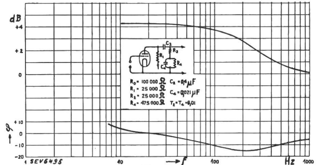
Fig. 9. Unkorrigierte Verstärkerstufe.
