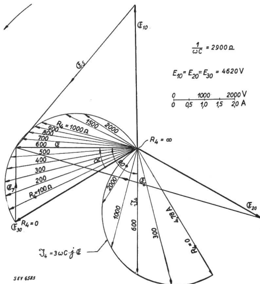
Fig. 5. Direkter Erdschluss über ohmschen Widerstand. Ortskurve der Spitzen von \mathcal{E} und \mathcal{I}_4 .
