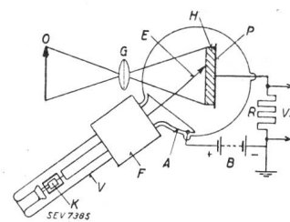
Fig. 1. Halbleiter-Bildabtaströhre. O Objekt, G Glaslinse. H Halbleiterschicht, P Metallplatte, F Magnetische Ablenkspulen, E Abtastelektronenstrahl, K Kathode, V Glaswand der Vakuumröhre, V_s Zum Verstärker, A Anode, B Batterie (Plattenspannung u_p ), R Eingangswiderstand des Verstärkers.
